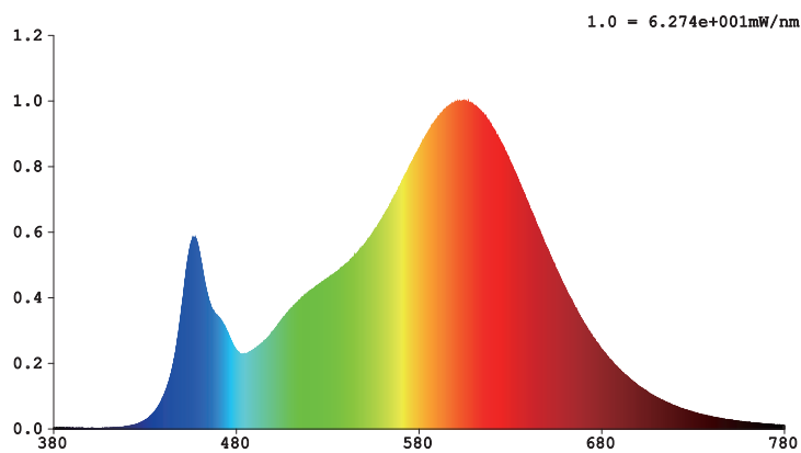
Spettroa ssoluto
