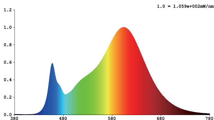
Spettro assoluto
