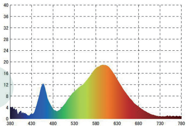
Spettro assoluto
