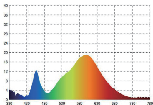
Spettro assoluto
